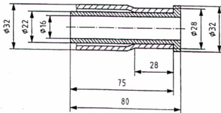
Hình B.4- Bộ phận giới hạn
