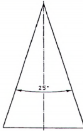
Hình 5 - Khuôn mẫu cho thử nghiệm bồn tiểu nam không có vành
