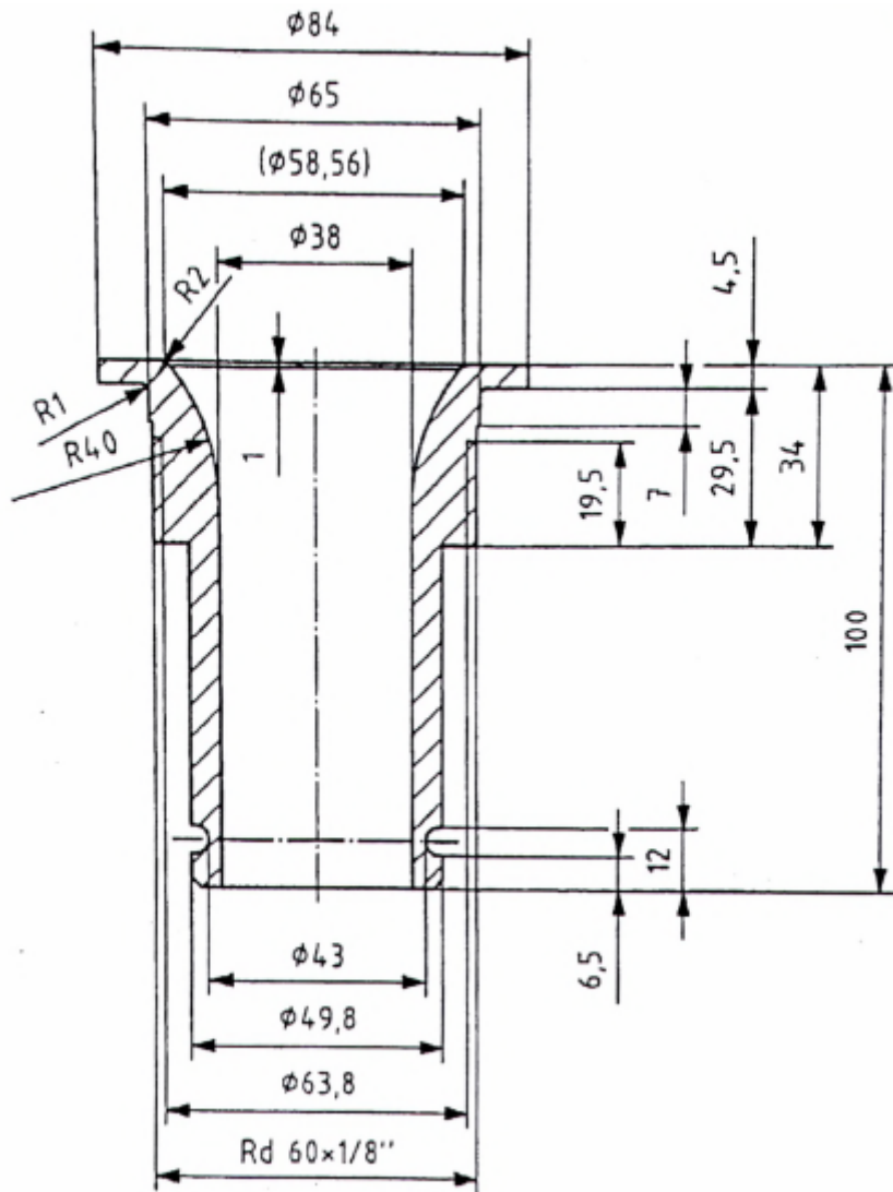
Hình B.3 - Thử nghiệm kết xả thoát với kết nối gắn liền đường ống xả
